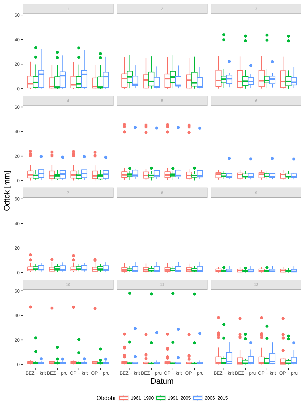
Obrázek 20: Měsíční odtokové výšky za období 1961-1990, 1991-2005 a 2006-2015 ve formě boxplotů bez opatření (BEZ) a s opatřením (OP)
