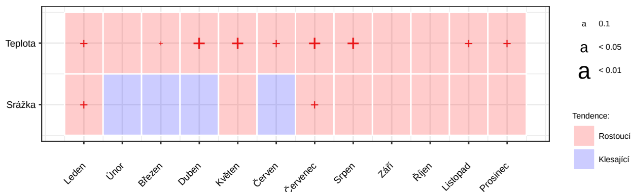
Obrázek 16: Analýza trendů srážek a teplot vzduchu pomocí Mann-Kendall testu
