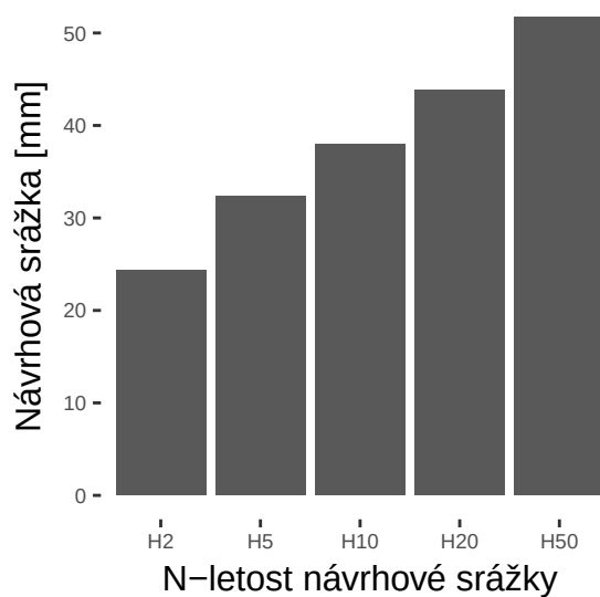
Obrázek 13: Návrhové srážky s dobou opakování 2, 5, 10, 20 a 50 let
