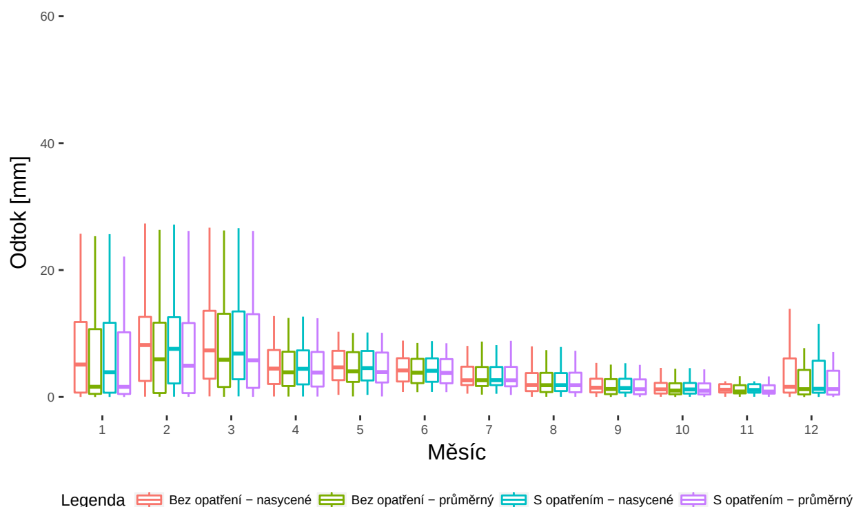
Obrázek 18: Průměrné měsíční odtokové výšky ve formě boxplotů pro jednotlivé varianty hodnocení
