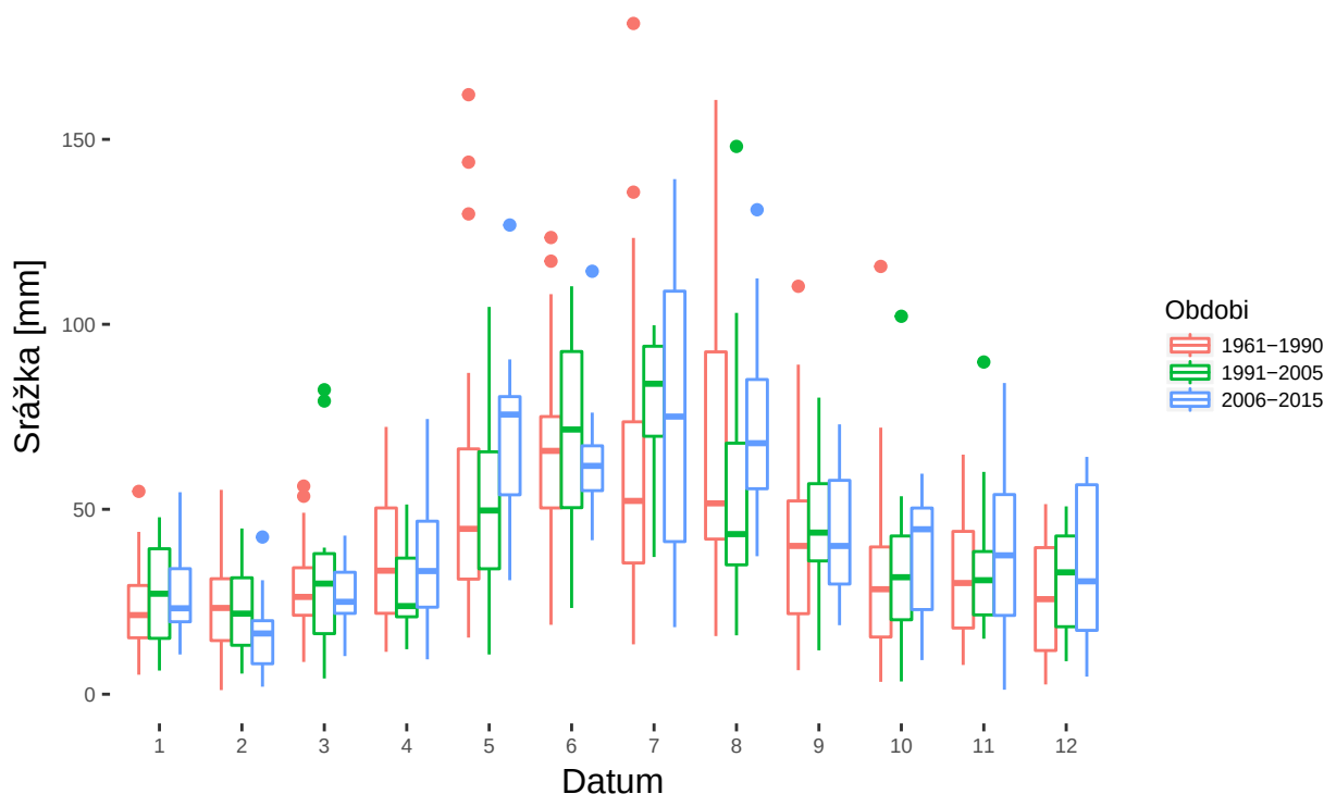
Obrázek 11: Měsíční srážkové úhrny za období 1961-1990, 1991-2005 a 2006-2015 ve formě boxplotů
