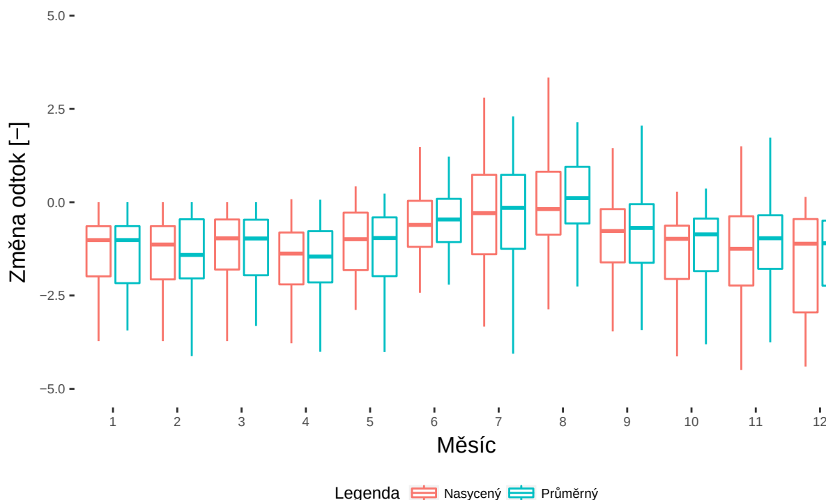
Obrázek 19: Změny měsíčních odtokových výšek ve formě boxplotů (pře opatřeními a po realizaci opatření)
