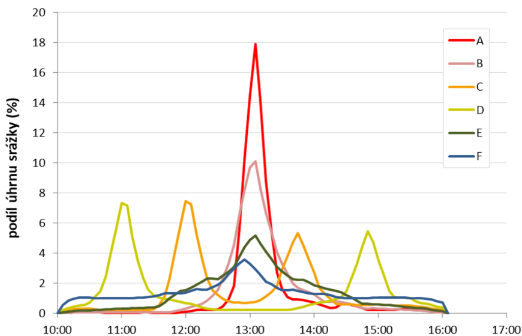
Obrázek 14: Průběh 5-min intenzit návrhových srážek
