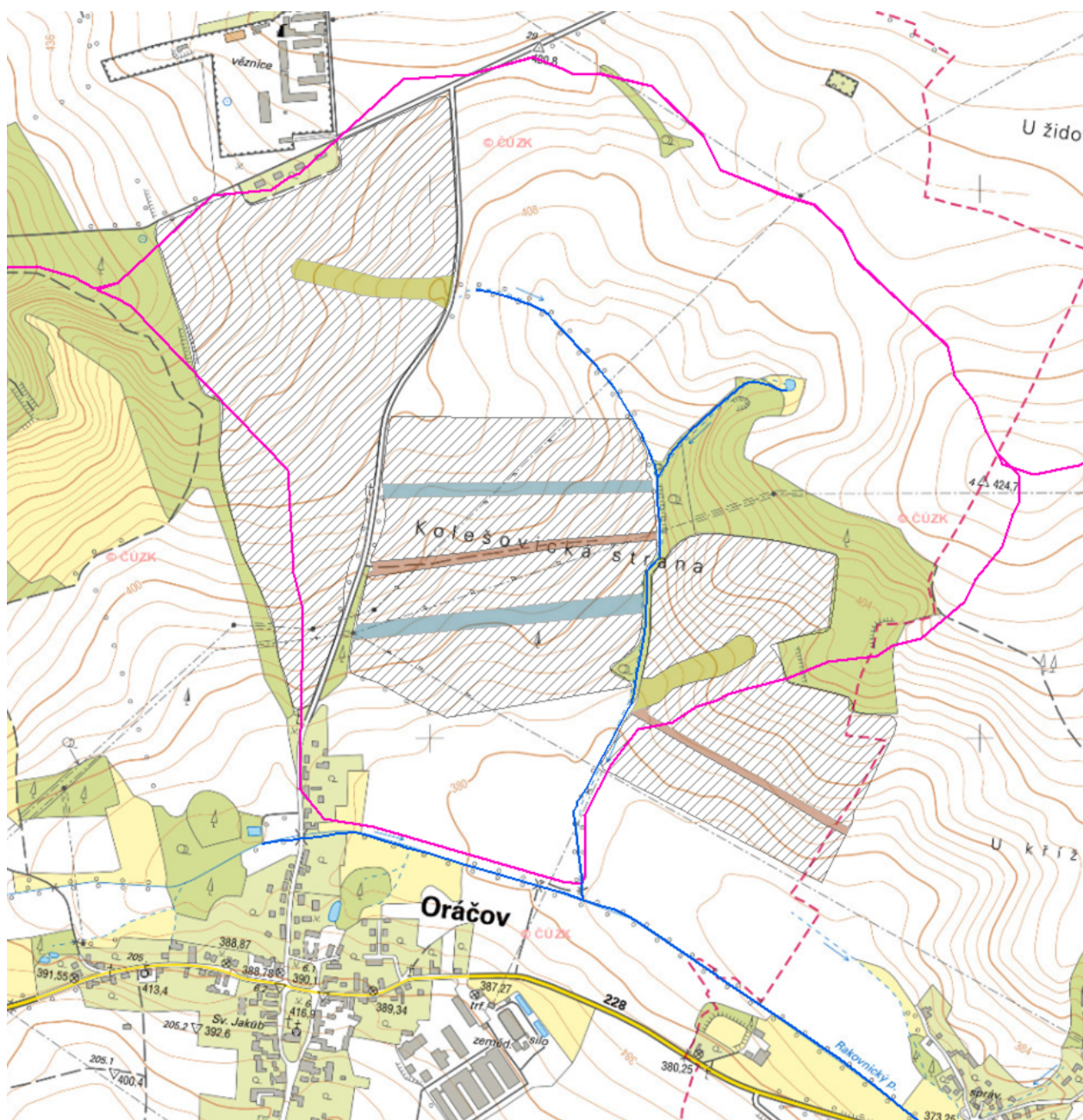
Obrázek 6: Lokalizace navržených protierozních opatření v povodí bezejmenného levostranného přítoku Rakovnického potoka
