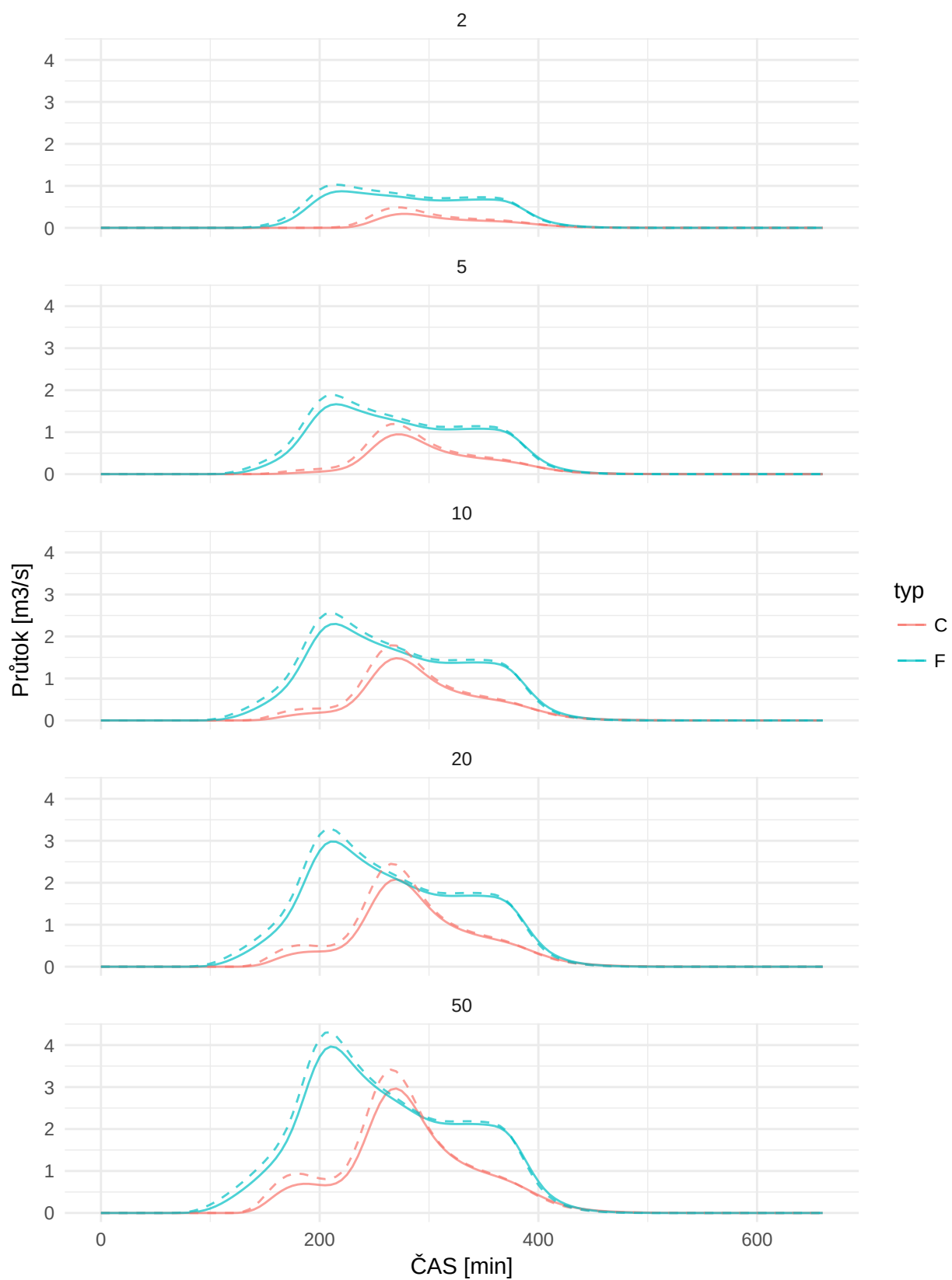
Obrázek 21: Návrhové průtoky dle N - letostí pro jednotlivé typy vln (čárkovaně-před opatřením, plně-po opatření)
