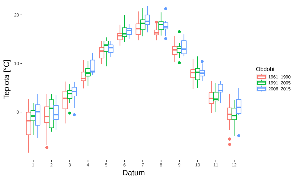
Obrázek 12: Průměrné měsíční teploty vzduchu za období 1961-1990, 1991-2005 a 2006-2015 ve formě boxplotů
