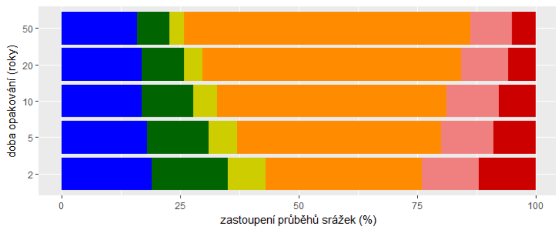
Obrázek 15: Rozdělení jednotlivých typů návrhové srážky
