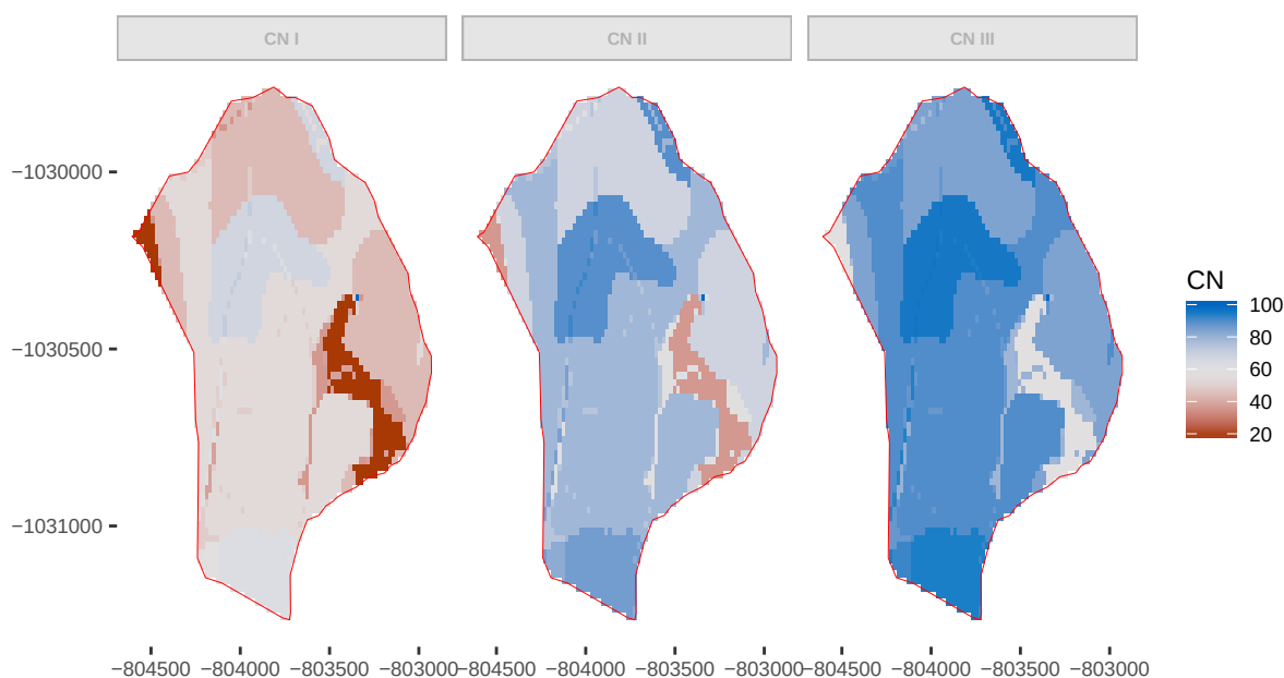
Obrázek 17: Hodnoty CN pro zájmové území a různé vláhové podmínky
