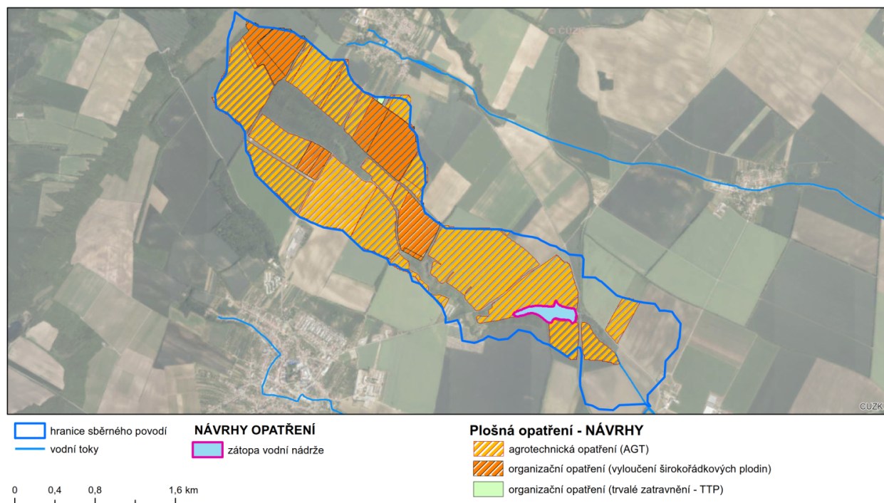
Obrázek 3: Navržená společná zařízení na ortofoto (Zdroj: ČÚZK)
